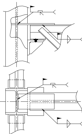
DETALLE 4
