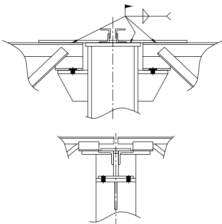
DETALLE 3
