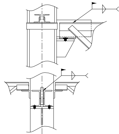
DETALLE 5
