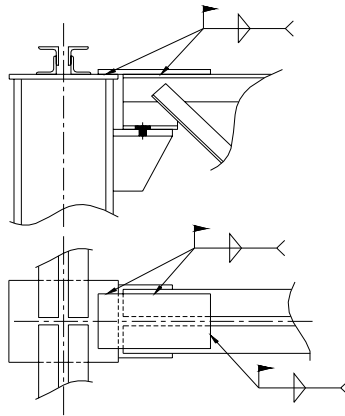
DETALLE 1
