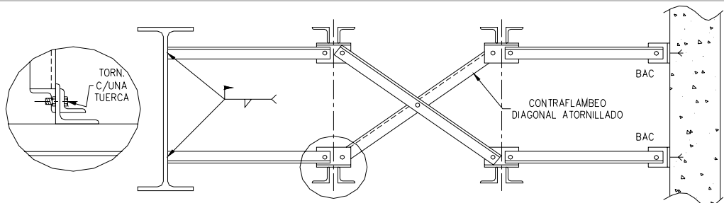
CONTRAFLAMBEO DIAGONAL ATORNILLADO
