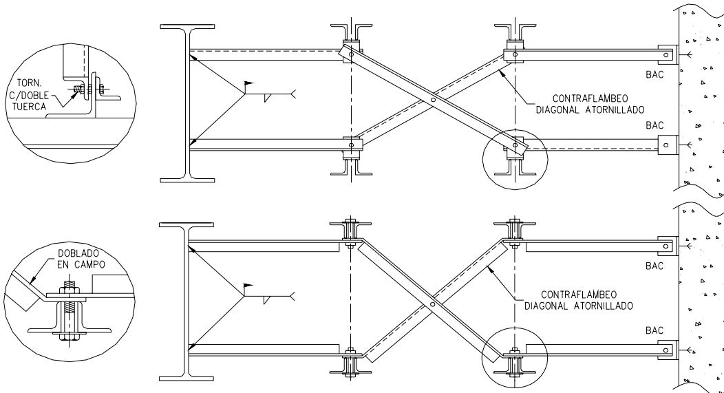
CONTRAFLAMBEO DIAGONAL ATORNILLADO
