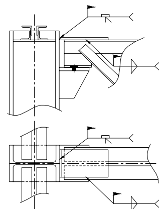
DETALLE 2
